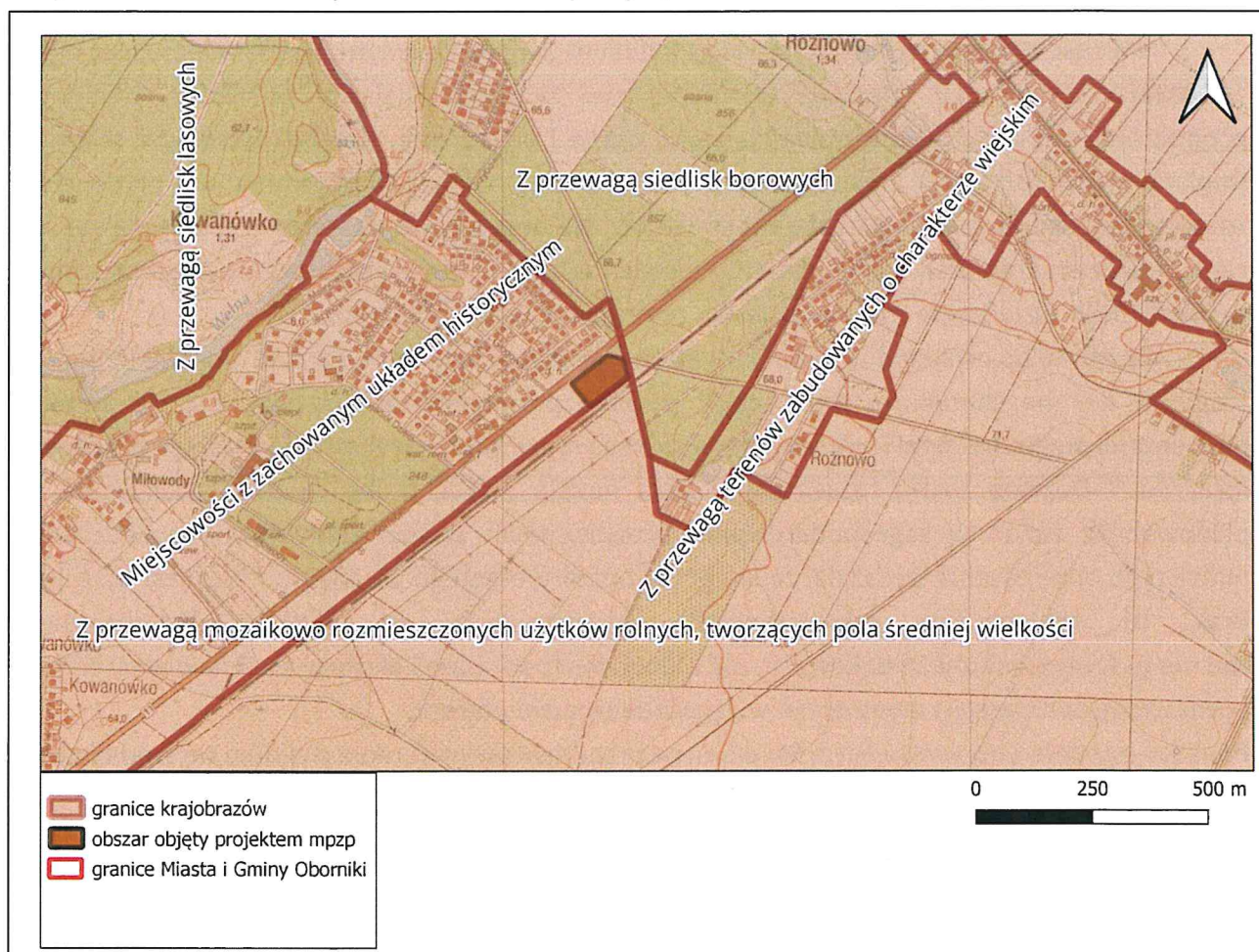
Mapa 5. Położenie obszaru objętego projektem mpzp granic krajobrazów.
