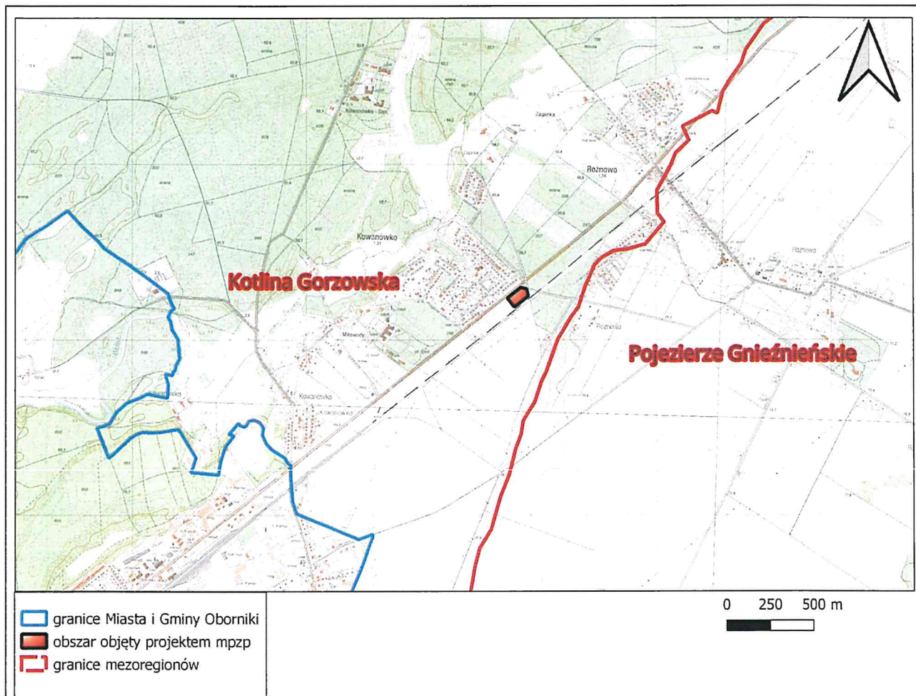
Mapa 2. Położenie obszaru objętego projektem mpzp na tle mezoregionów.
